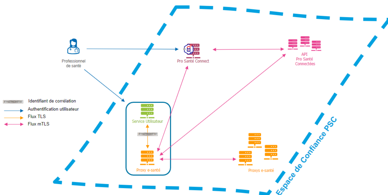
Figure 5 - Principaux échanges au sein de l'espace de confiance
