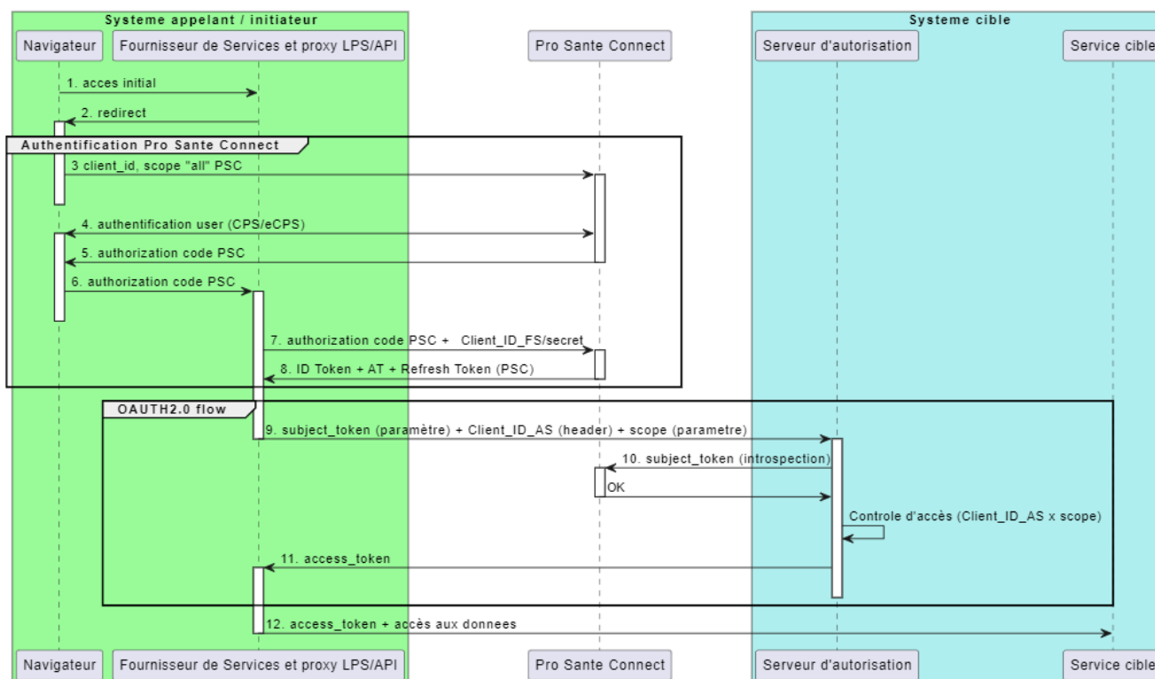
Figure 4 - Diagramme de séquence d'un appel d'une API Pro Santé Connectée
