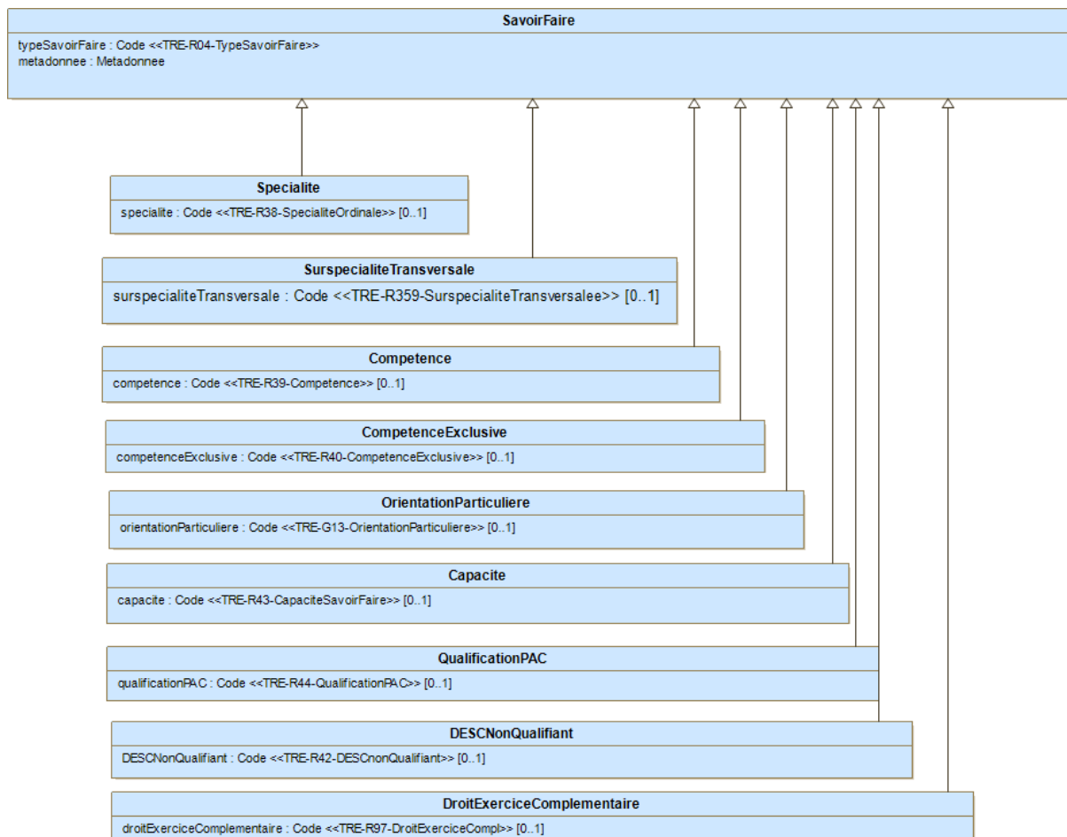
Figure 9 SavoirFaire
