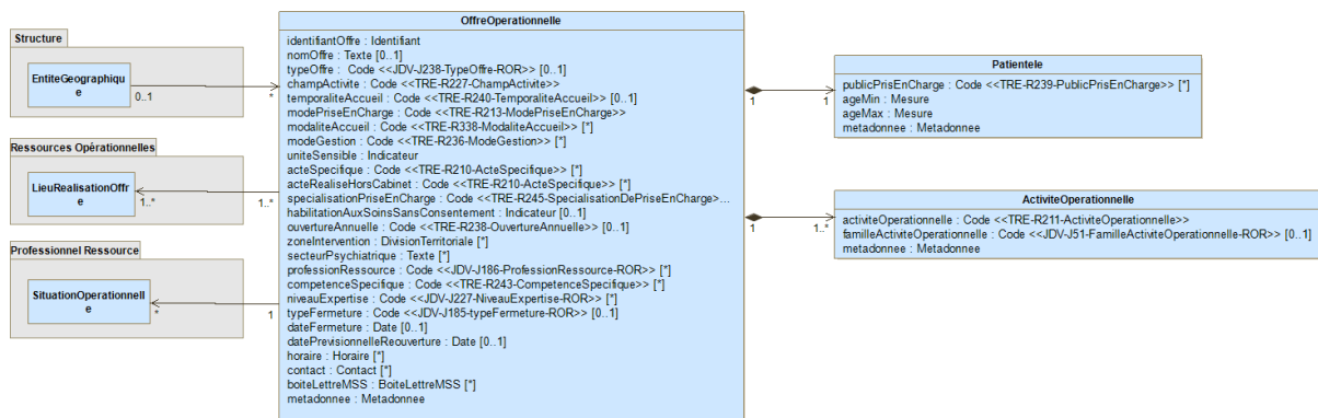
Figure 6 Offre Opérationnelle
